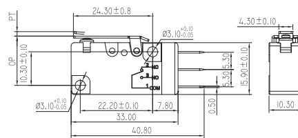
KW7F-5T-□□
