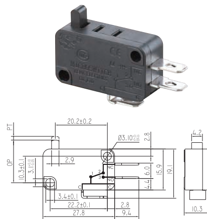
KW7-11-□□
