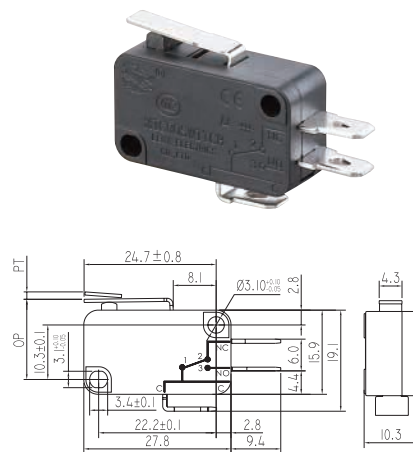
KW7-32L-□□
