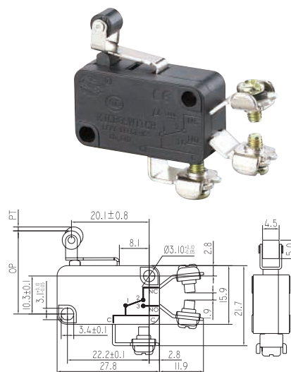
KW7-32L-□□
