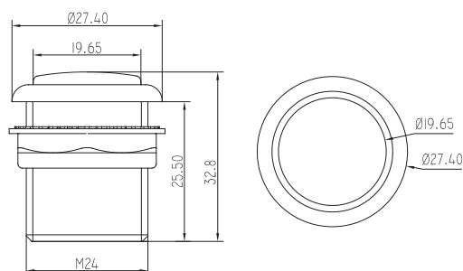
PBS – 010 Y □
