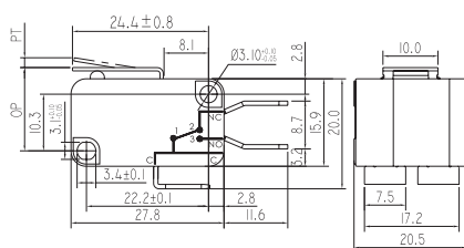
KW7-DU-□□
