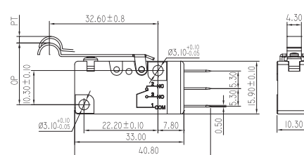
KW7F-1L-□□
