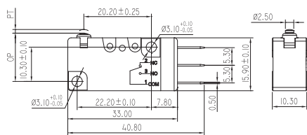
KW7F-2T-□□
