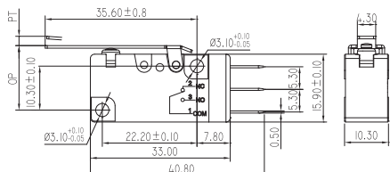
KW7F-3T-□□
