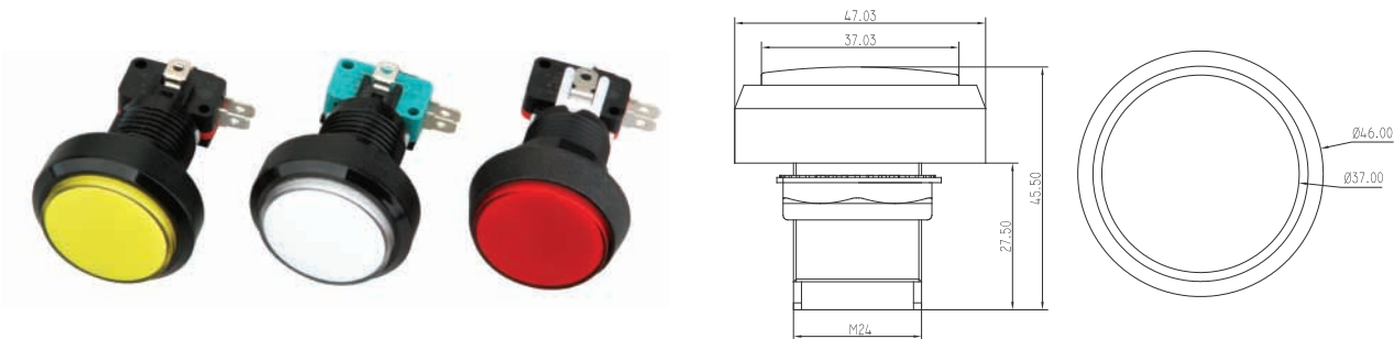
PBS – 005 Y
