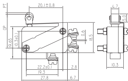
KW7-7-□□
