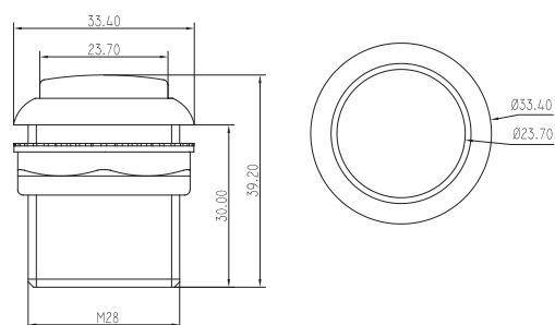
PBS – 010 Y □
