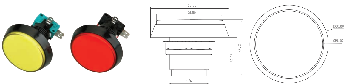
PBS – 006 Y
