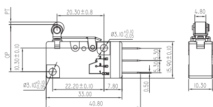
KW7F-0L-□□
