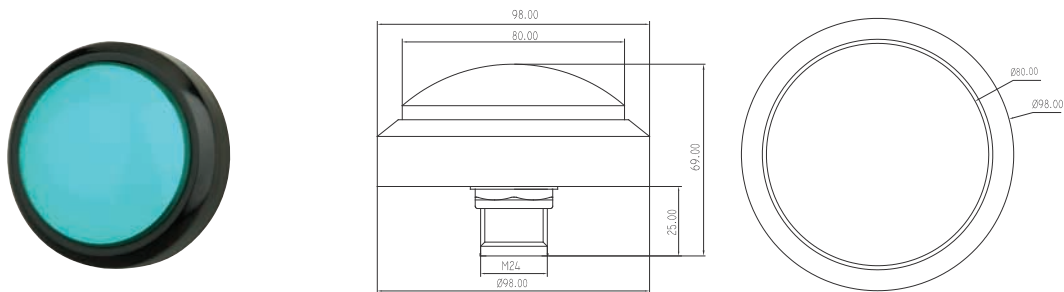
PBS – 006 Y
