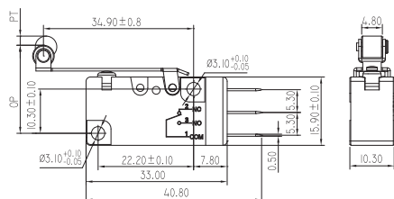
KW7F-9T-□□
