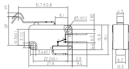
KW7-9-□□
